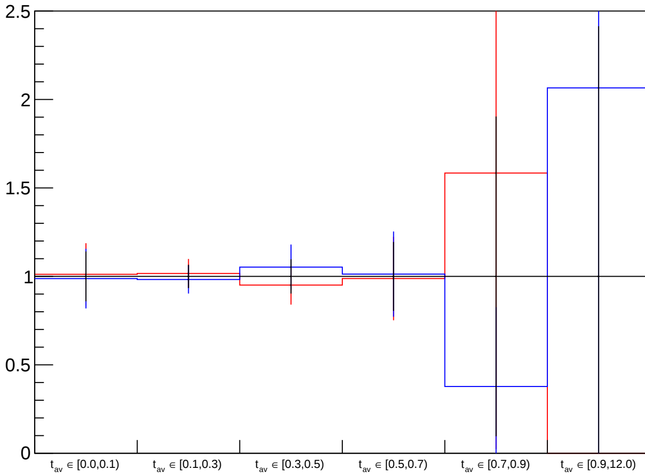
Pseudo-ex background ratio, \rho \in [320, 440)
